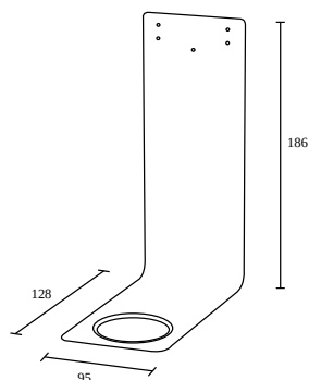
Tropfschale NSU 2-5-11-12
